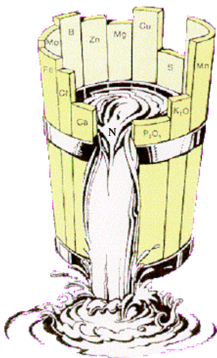
Figure 36 : Le tonneau de Liebig, illustration de la loi du facteur limitant ou loi du minimum
