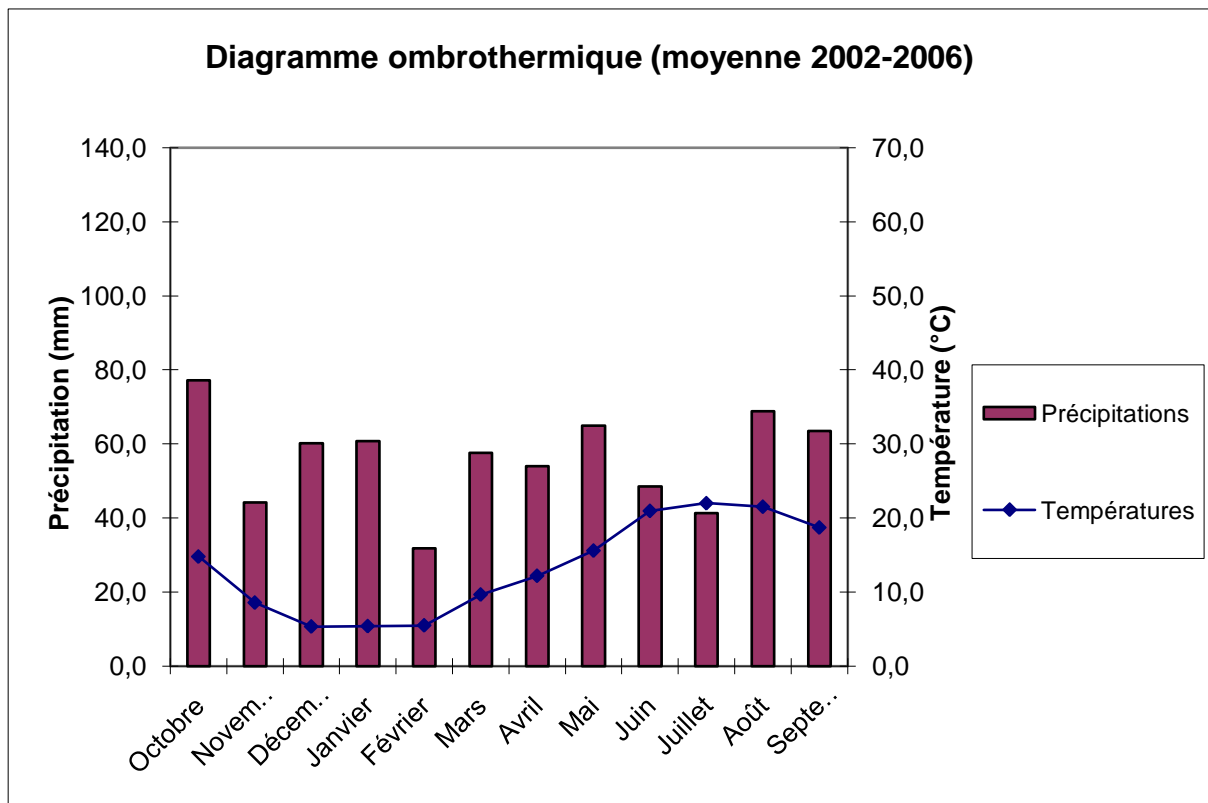
Figure 8 : Précipitations et températures moyennes sur la période 2002-2006
