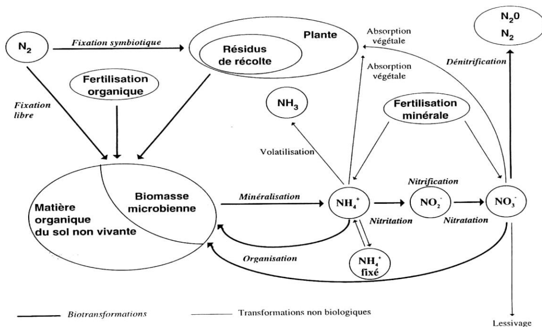
Figure 2 : Transformations biologiques et non biologiques affectant le devenir de l'azote dans les sols. Source : Nicolardo et al., 1996.
