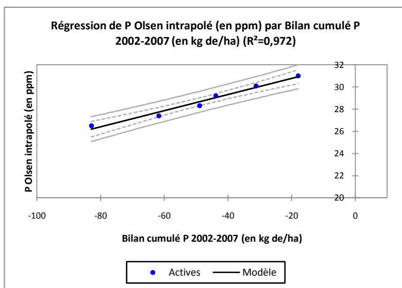
Figure 26 : régression entre le bilan P exporté cumulé et le P Olsen intrapolé.
